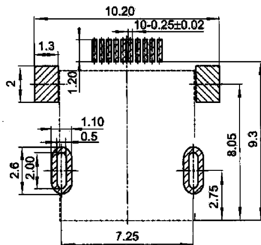
印制线路板推荐开孔尺寸
