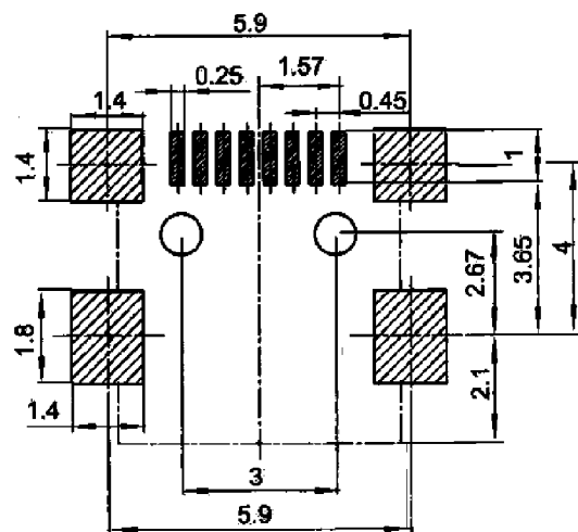
印制线路板推荐开孔尺寸
