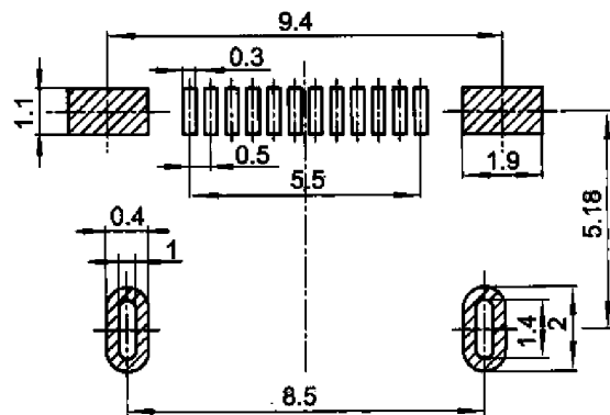
印制线路板推荐开孔尺寸
