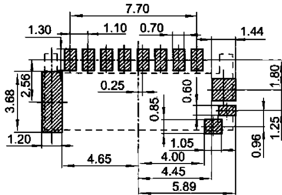
印制线路板推荐开孔尺寸
