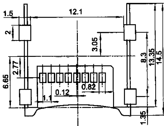
印制线路板推荐开孔尺寸
