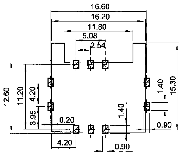
印制线路板推荐开孔尺寸
