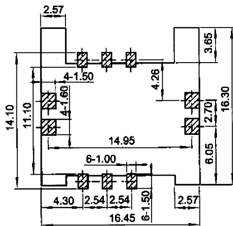
印制线路板推荐开孔尺寸
