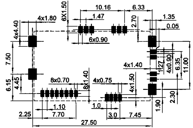
印制线路板推荐开孔尺寸
