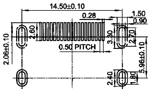
印制线路板推荐开孔尺寸
